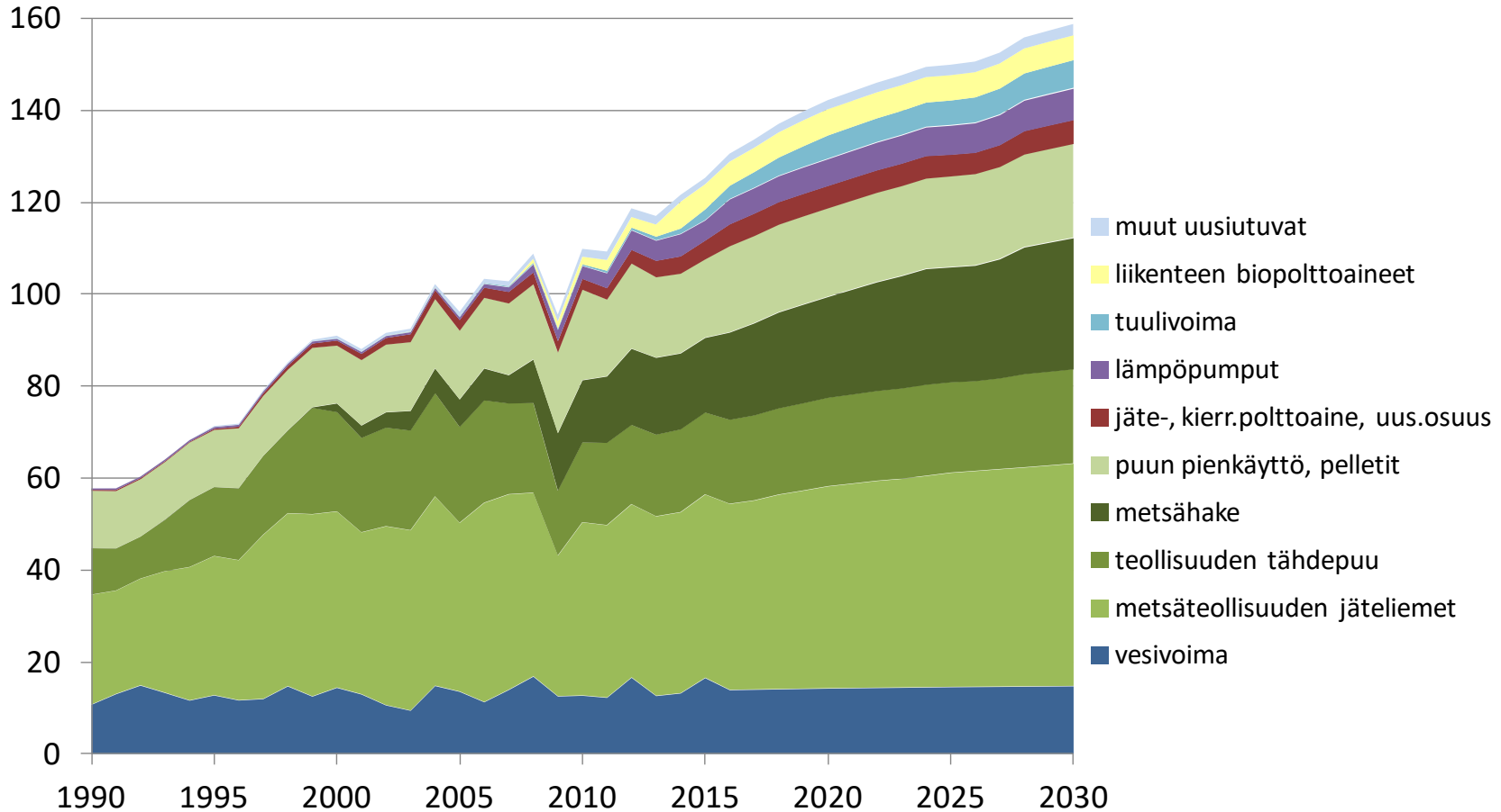
UUSIUTUVA ENERGIA, TWh
