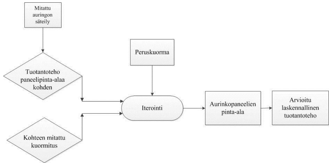
Kuva 7.3 Paneelipinta-alan laskeminen aurinkoisuuskertoimen avulla
