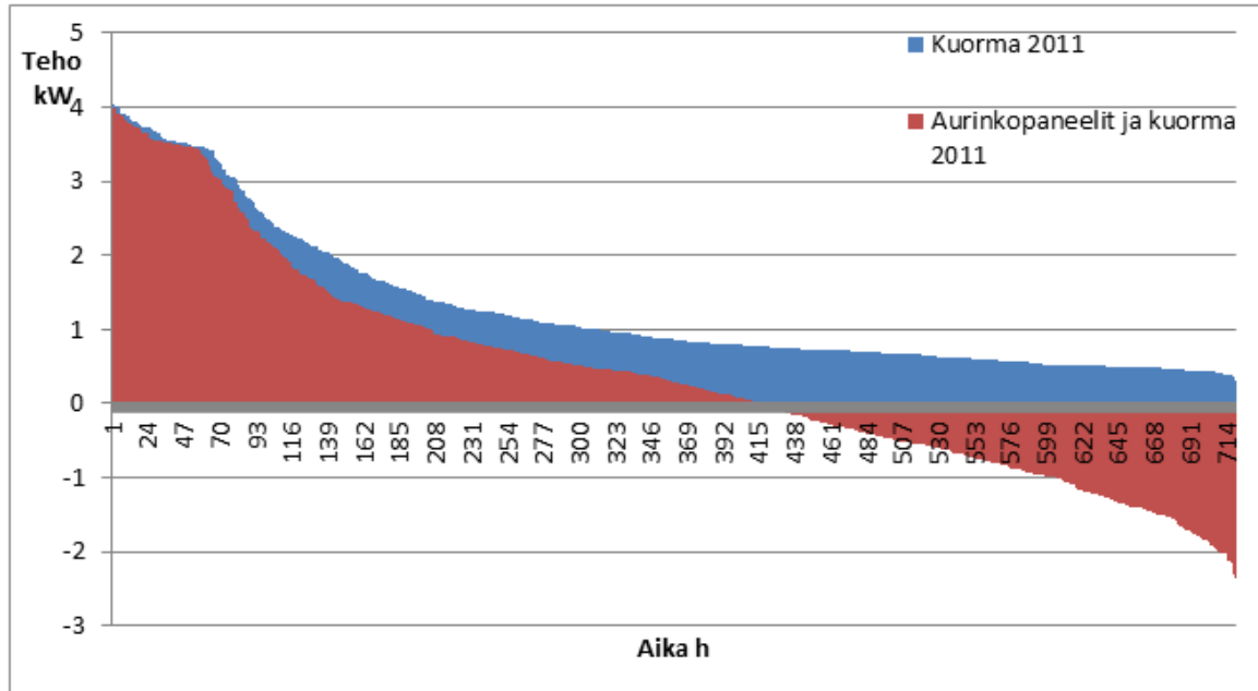
Kuva 6.4 Kesäkuun pysyvyysskäyrä
