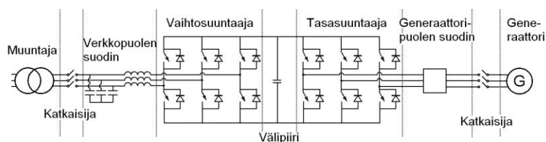
Kuva 8. Back-to-back täystehokonvertterilla varustetun tuulivoimalan piirikaavio.
