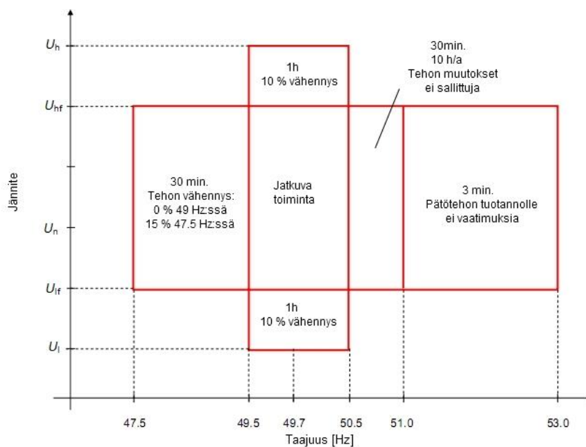
Kuva 16. Tuulivoimalan toiminta-alueet eri jännitteillä ja taajuuksilla Tanskassa yli 100 kV jännitteillä. (DEN 2004b)
