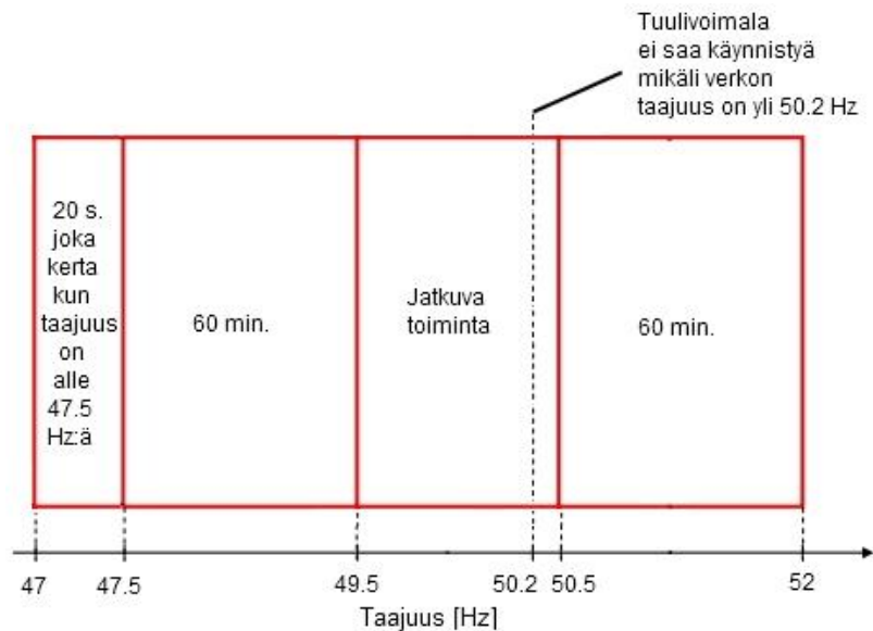
Kuva 20. Tuulipuistoille asetetut verkkomääräykset taajuuden suhteen Irlannissa. (IRE 2009)
