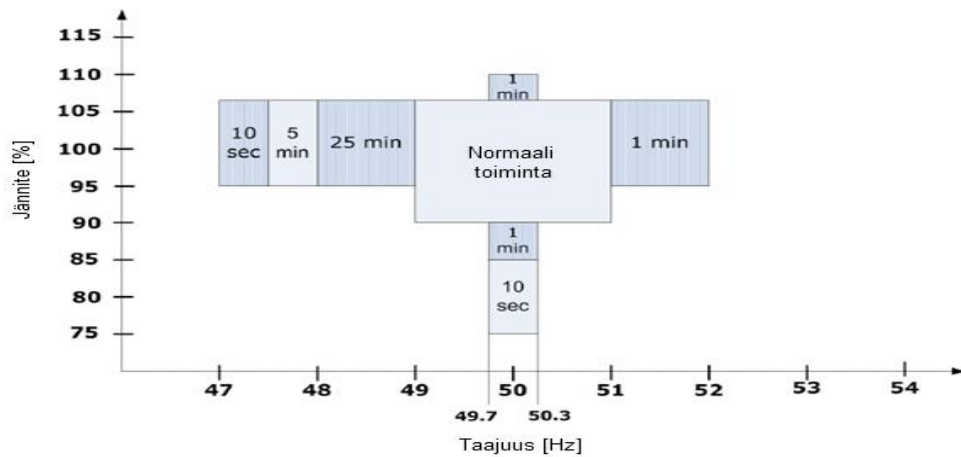
Kuva 17. Tuulivoimalan toiminta-alueet eri jännitteillä ja taajuuksilla Tanskassa alle 100 kV jännitteillä. (DEN 2004a)
