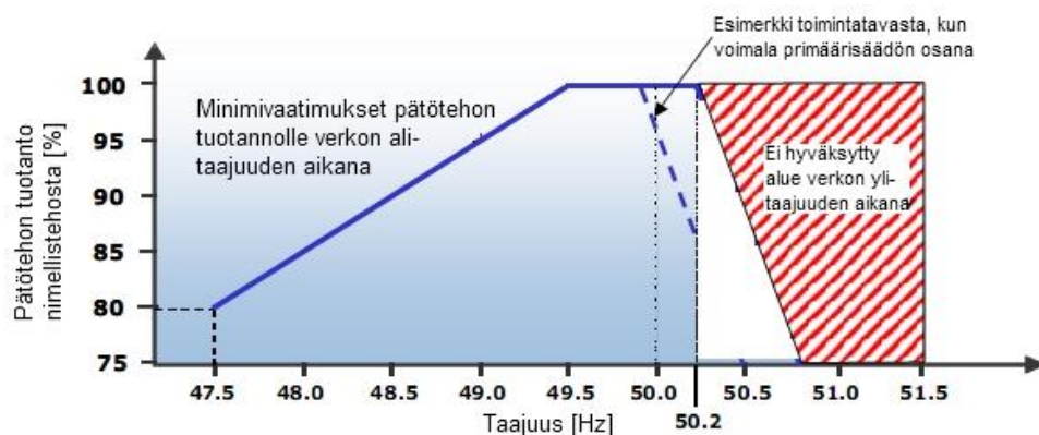
Kuva 24. Saksan verkkomääräys tuulivoimaloiden verkkoon syötetyn pätötehon vaaditusta rajoittamisesta ja sen sallitulle laskulle taajuuden funktiona. (GER 2007)
