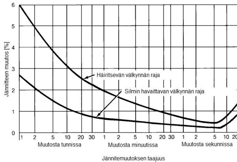
Kuva 11. Välkynnän taajuuden vaikutus havaittavuuteen ja häiritsevyyteen. (IEEE 1993)
