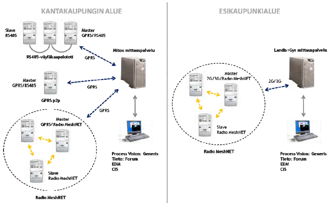
Kuva 4. Etäluennan tekninen toteutus Helsingin kantakaupungin ja esikaupungin alueilla
