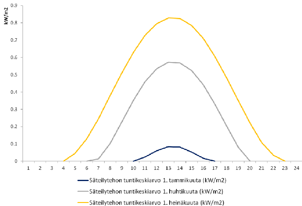
Kuva 30. Vaakatasoon asennetun aurinkopaneelin vuorokauden neliometrikohtaiset teoreettiset säteilytehon tuntikeskiarvot ( \text{kW/m}^2 ) tammikuussa, huhtikuussa ja heinäkuussa Helsinki-Vantaan lentoasemalla. (Lähde: Hannu-Pekka Hellman, Aalto-yliopiston sähkötekniikan korkeakoulu)
